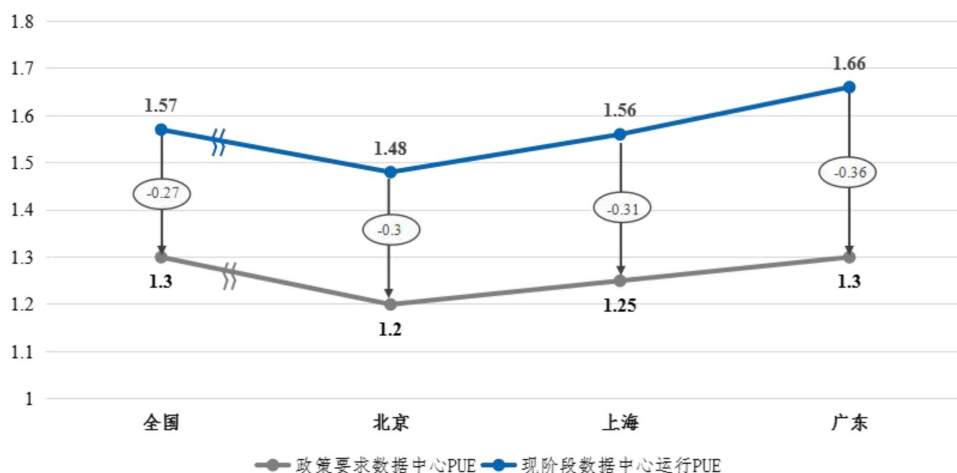
图3：2022 年数据中心实际 PUE 与政策要求 PUE 差异比较
