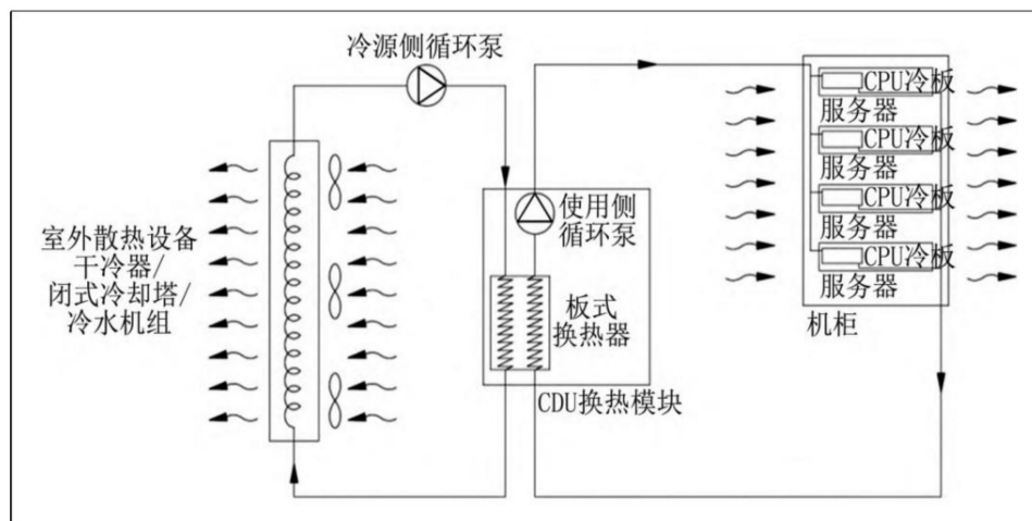
图5：冷板式液冷原理示意图
