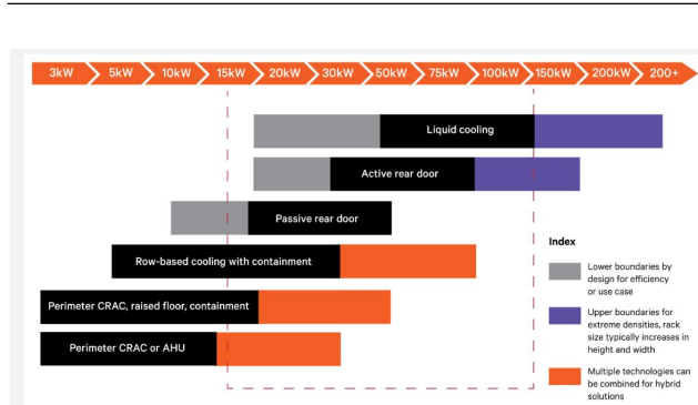
图2：单机柜功率密度与冷却方式演变
